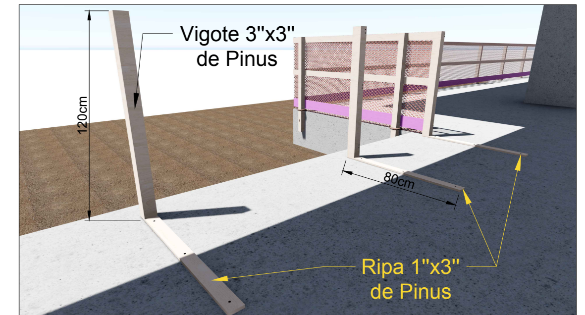
2ª ETAPA: REVISTA O VIGOTE NO VERGALHÃO CHUMBADO NO PISO
