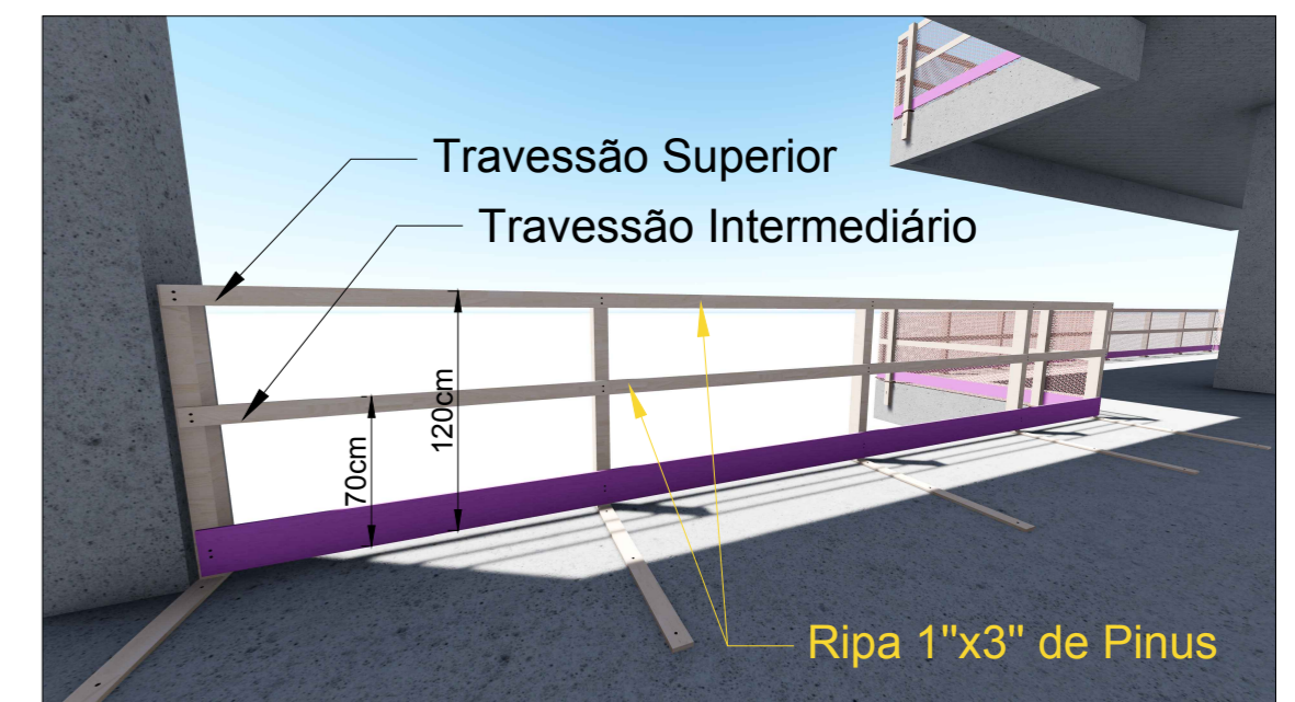
4ª ETAPA: PREGUE OS TRAVESSÕES INTERMEDIÁRIOS E SUPERIORES SEMPRE RESPEITANDO O DISTANCIAMENTO CORRETO OBS: ESTE GUARDA CORPO SOFRERÁ ALTERAÇÕES EM SUA ALTURA DEVIDO A RIPA INSTALADA EMBAIXO DO VIGOTE CONFORME DETALHA A IMAGEM DA 1ª ETAPA
