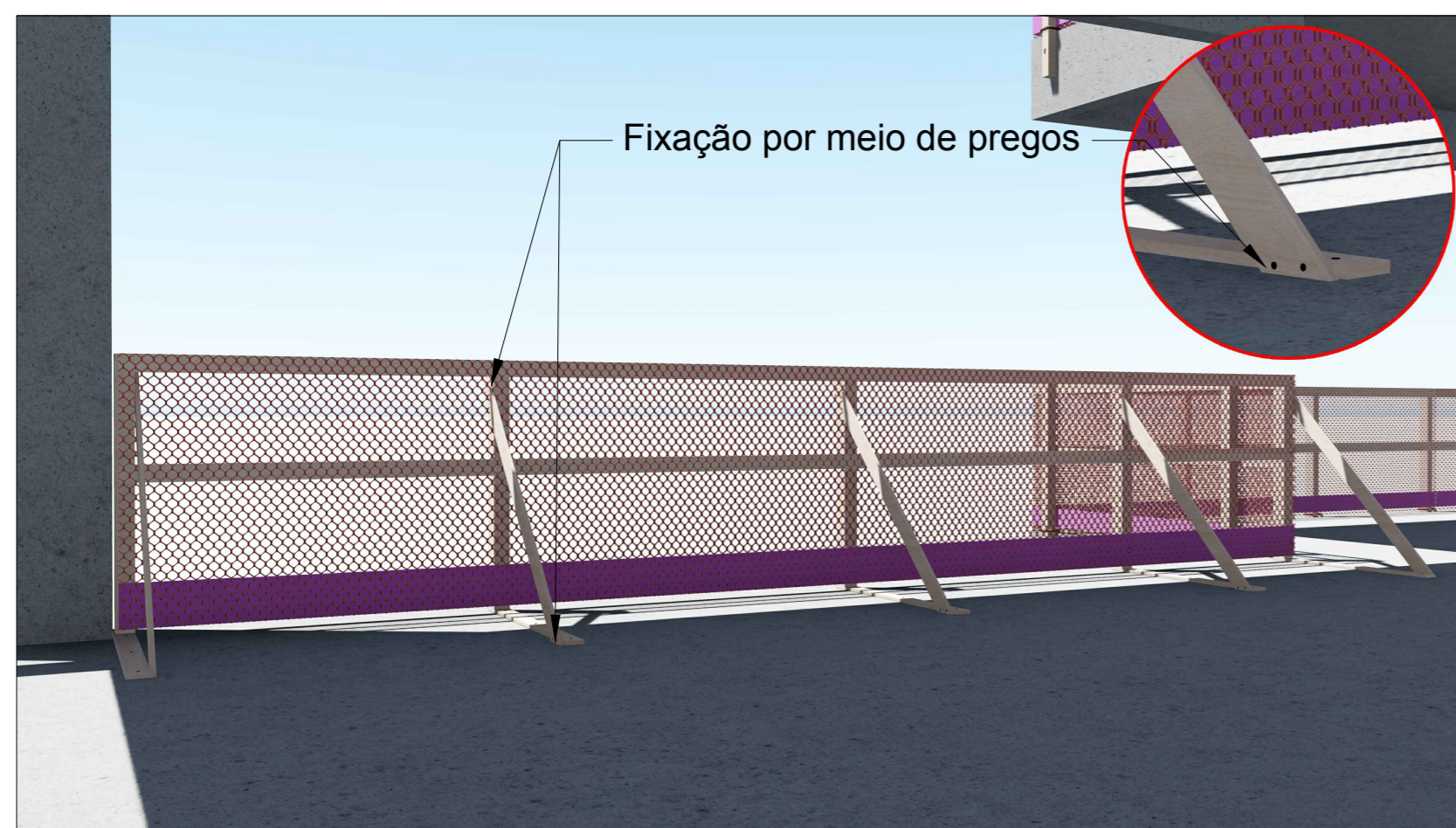
5ª ETAPA: FINALIZE O SISTEMA INSTALANDO A MÃO FRANCESA, NESTE PROCESSO É NECESSÁRIO QUE A TELA DE PROTEÇÃO SEJA CORTADA NO LOCAL ONDE A RIPA DEVERÁ PASSAR PARA QUE POSSA SER FIXADA NO MONTANTE
