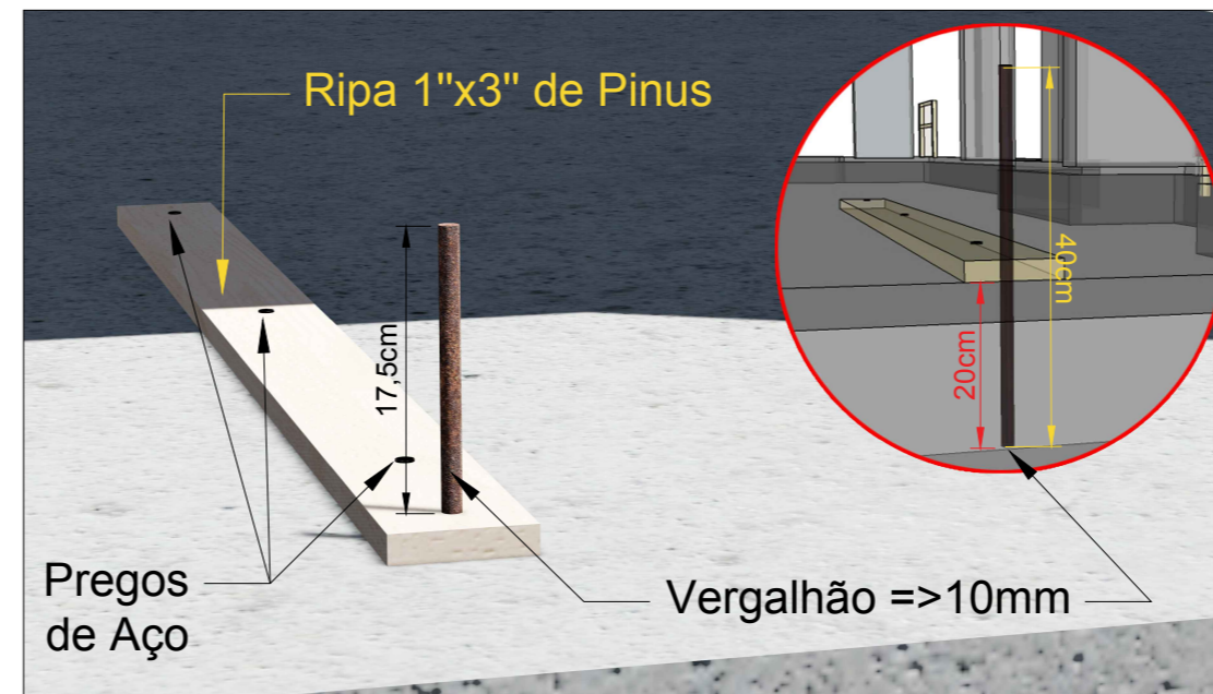
1ª ETAPA: INSTALAR OS VERGALHÕES A UMA DISTÂNCIA \leq 1,5m CHUMBANDO OS NO PISO POR MEIO DE CHUMBADORES QUIMICOS, APÓS FURE A RIPA E ENCAIXE NO VERGALHÃO CHUMBADO
