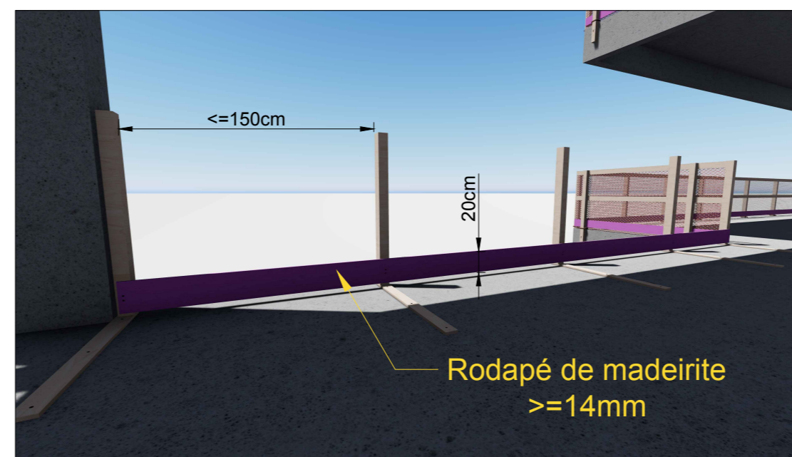
3ª ETAPA: INSTALE OS RODAPÉS DE MADEIRITE POR MEIO DE PREGOS NOS MONTANTES FIXADOS NO PISO
